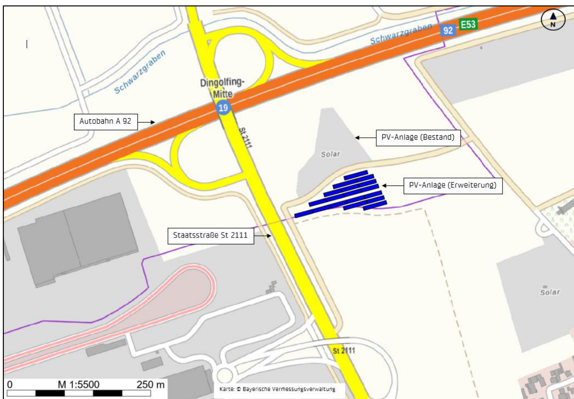
Abbildung 1: Lageplan und Immissionsorte
