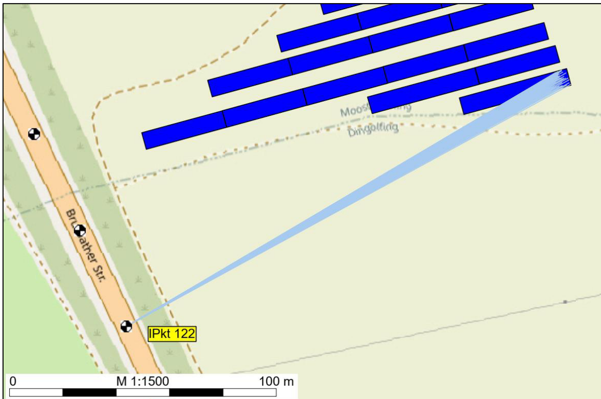
Abbildung 3: Darstellung der Reflexionen auf IPkt 122
